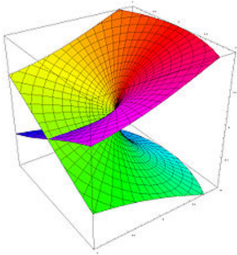
Superficie de Riemann de \sqrt{z}
