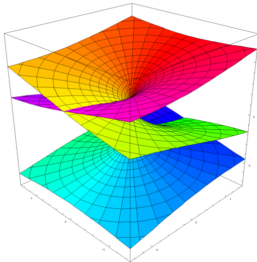
Superficie de Riemann de \sqrt[3]{z}
